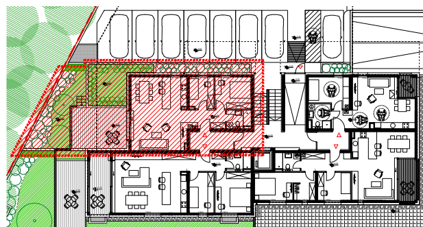
TLOCRT PRIZEMLJA
