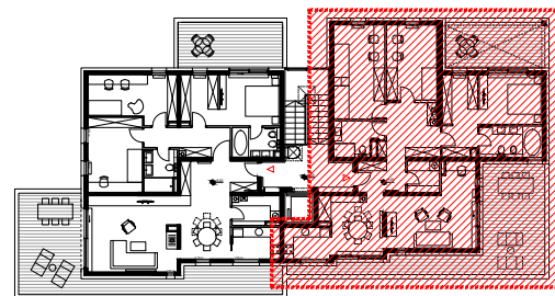
TLOCRT POTKROVLJA
