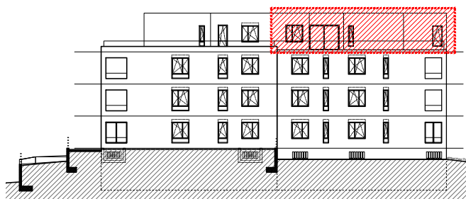
JUŽNO PROČELJE
