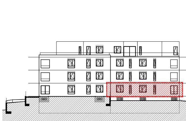
JUŽNO PROČELJE
