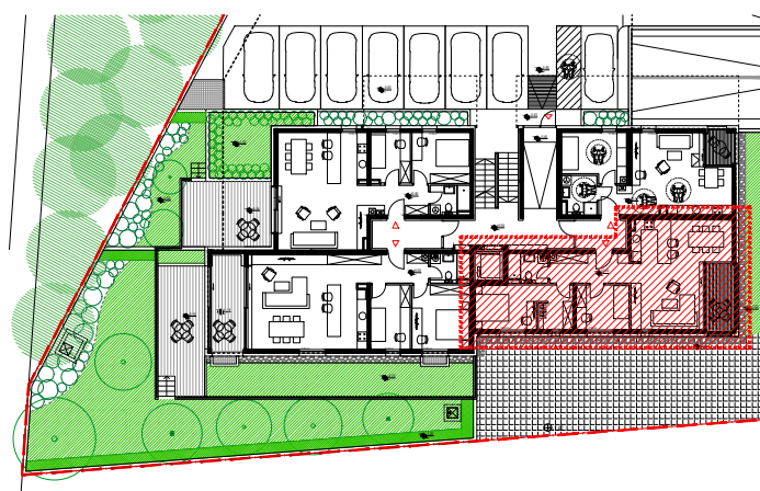
TLOCRT PRIZEMLJA
