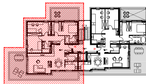
TLOCRT POTKROVLJA
